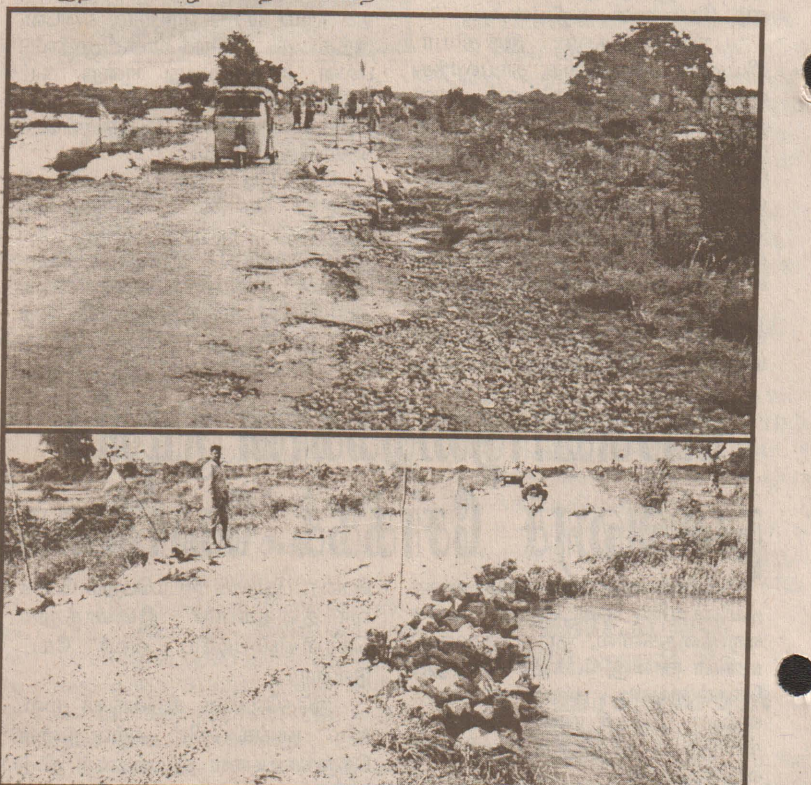
உமையாள்புரம் பகுதியில் வெள்ளத்தால் சேதமடைந்த ஏ-9 வீதி, தற்காலிகமாகச் செப்பனிடப்பட்டு போக்குவரத்துக்கு ஏற்பாடு செய்யப்பட்டுள்ளது. தற்காலிகமாகச் செப்பனிடப்பட்ட வீதி மற்றும் மதகிணைப் படங்களில் காணலாம்.
